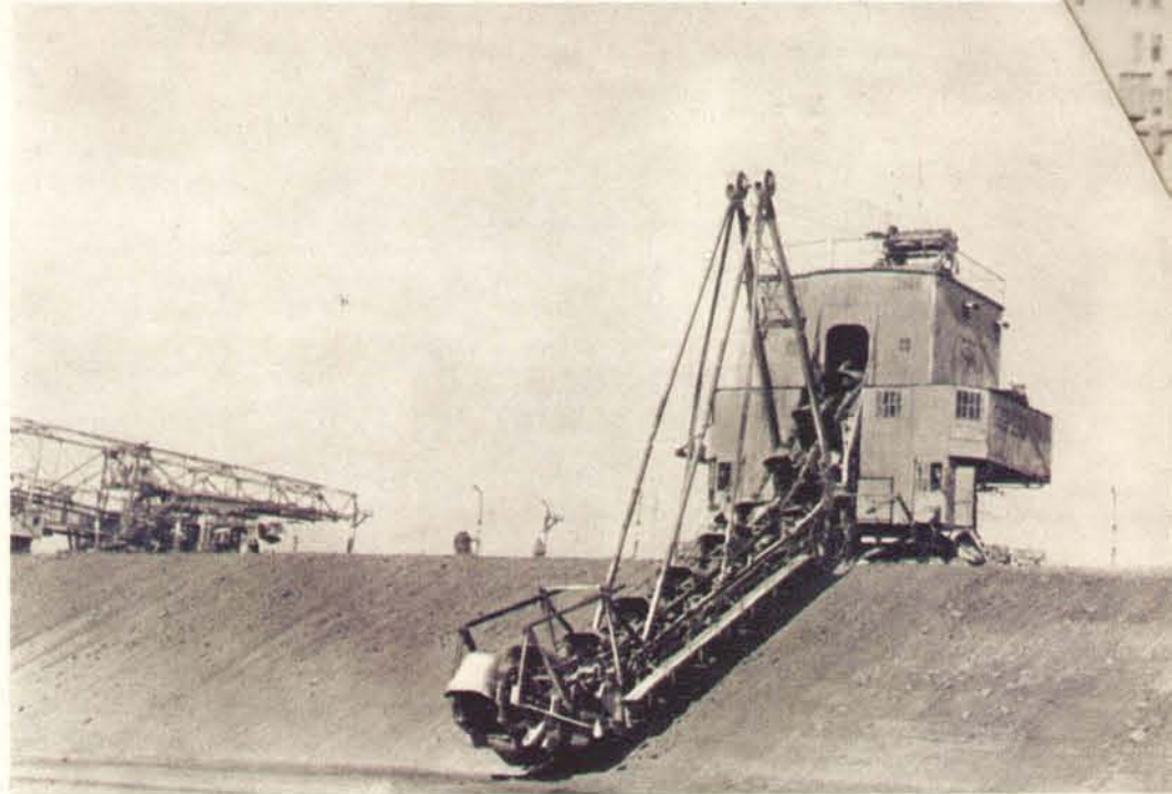
Камышбурунский железорудный комбинат (Крымская область) — одно из передовых предприятий Советской страны. Комбинат ежемесячно дает большое количество агломерата сверх плана. В марте коллектив предприятия работал еще упорней, еще производительней. Став на сталинскую трудовую вахту, передовые рабочие добиваются значительного перевыполнения производственных заданий. На снимке — один из многоковшовых экскаваторов Камышбурунского комбината в работе.
