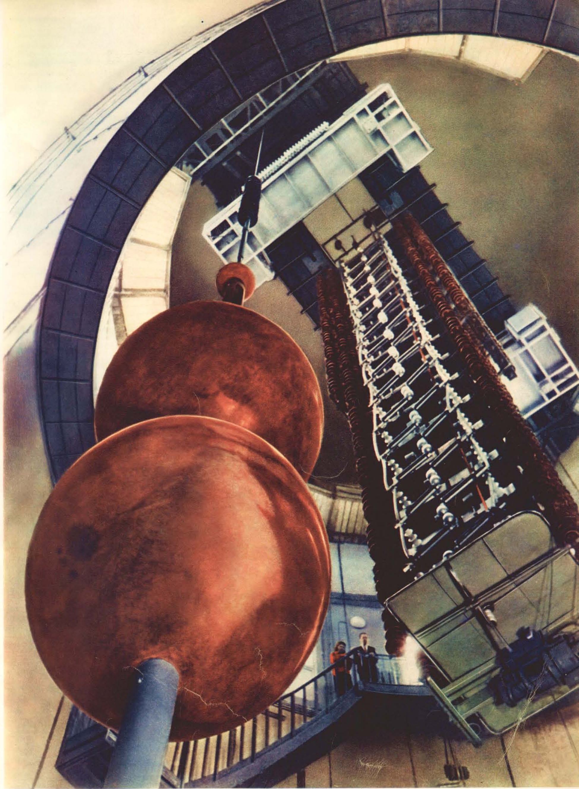
Решая проблемы сверхдальних передач электроэнергии с великих строек коммунизма, советские ученые производят сложнейшие опыты и внедряют в практику результаты своих исследований. Большое место в этой работе принадлежит лаборатории высоковольтного газового разряда Энергетического института имени Г. М. Кржижановского Академии наук СССР. На снимке — импульсный генератор напряжением в 3 000 000 вольт в лаборатории института.
