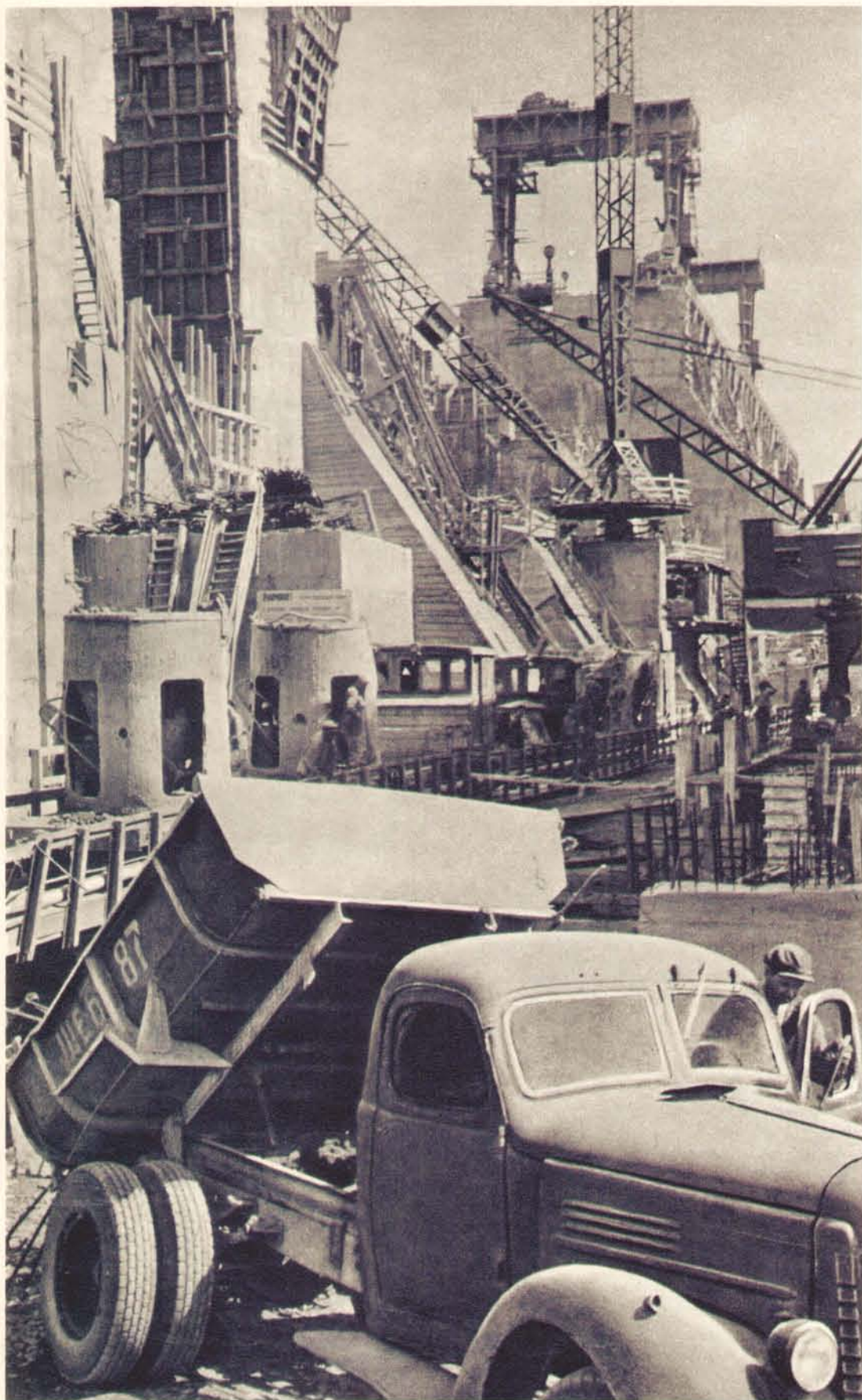
Бетонные работы на строительстве Усть-Каменогорской гидроэлектростанции.
