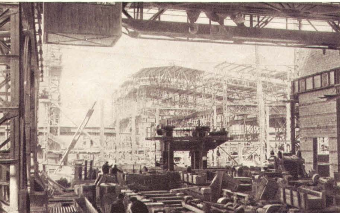
Кузнецкий комбинат — гигант современной металлургии. На снимке — сборка прокатного стана в дни строительства комбината.
