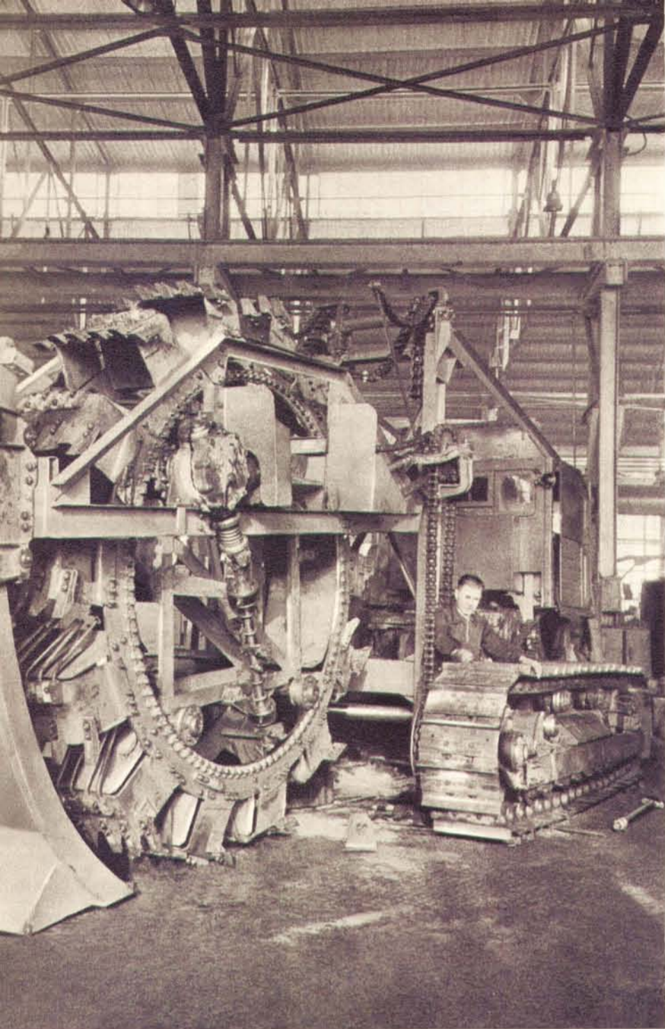
В СССР осуществляется широкая механизация тяжелых и трудоемких работ. Все больше машин и механизмов отправляют советские заводы в различные концы страны. На снимке — в цехе Дмитровского экскаваторного завода. Сборка колесно-гусеничного экскаватора для рытья мелких оросительных каналов.
